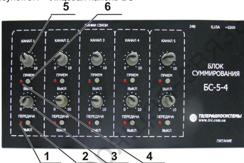
Рисунок 3.1 – Лицевая панель БС
